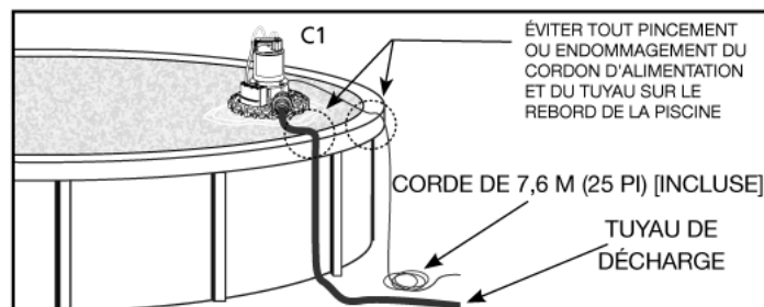
Figure C - Installation de pompe à tirer (vue latérale)
