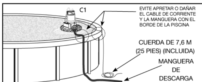
Figura C: Instalación desde un costado de la piscina (vista lateral)
