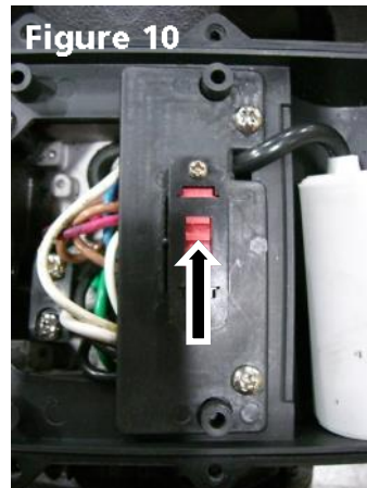
Figure 10 Pour passer au fonctionnement à 230 volts, faire glisser le commutateur de tension à la position « 230 » volts
